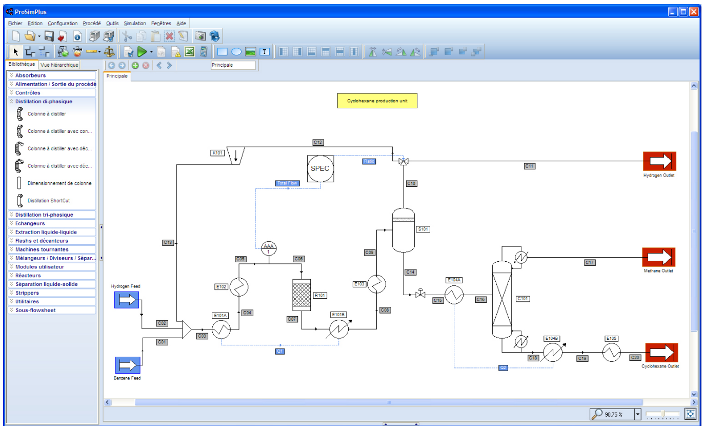
Schéma de l'unité de production de cyclohexane
