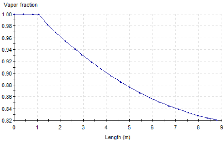
E107 - Mass vapor fraction
