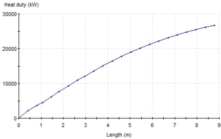
E107 - Heat duty
