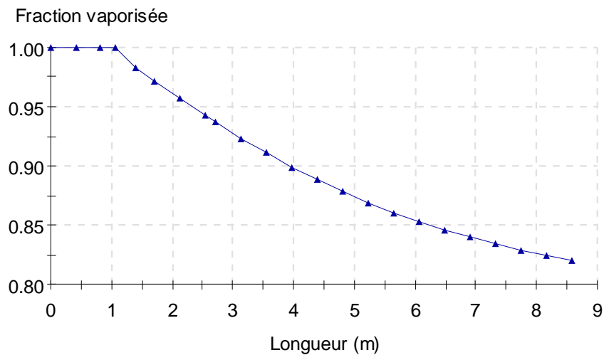
Profil de fraction vaporisée massique le long du condenseur
