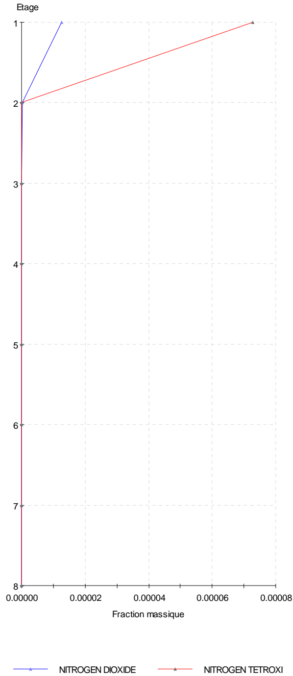
Profil des fractions massiques liquide dans la colonne
