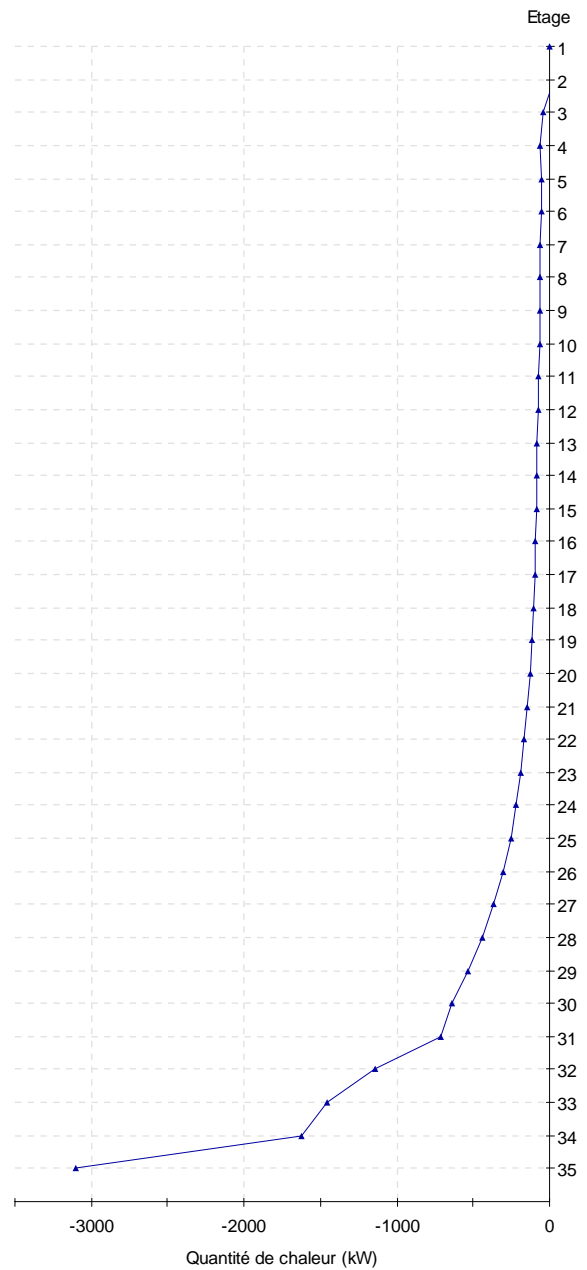
Profil de quantité de chaleur échangée dans la colonne
